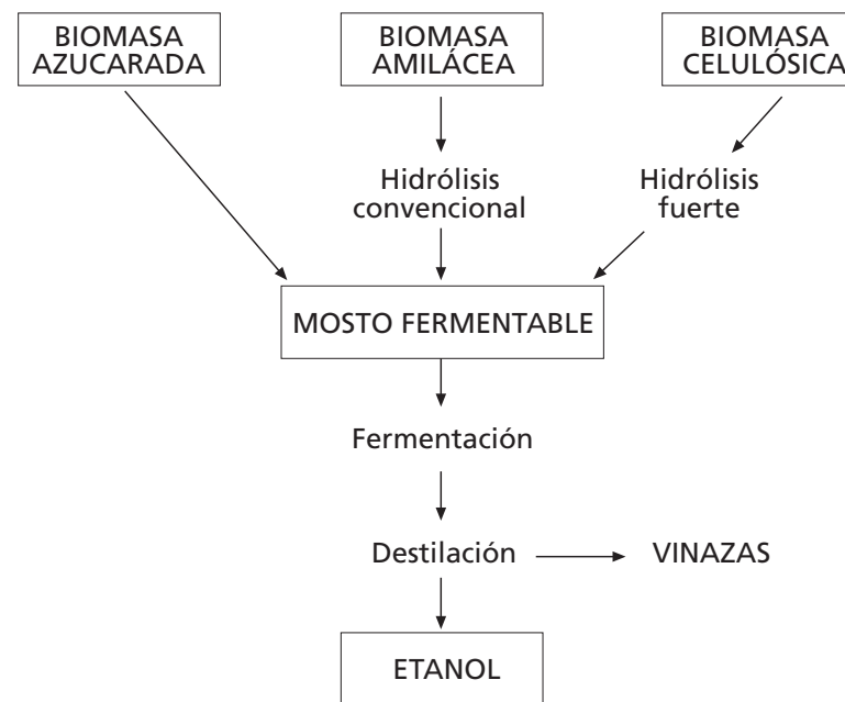
Vías de obtención del bio etanol por vía biológica.
